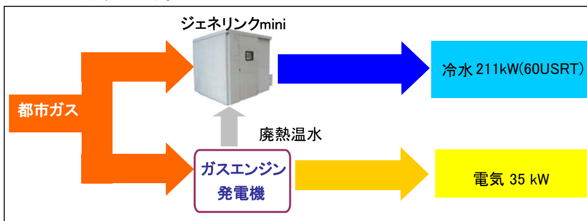
図 コージェネレーションシステムのフロー例 [211kW(60USRT)時]
